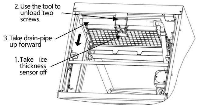
[SRM-105/125A/125UB]
