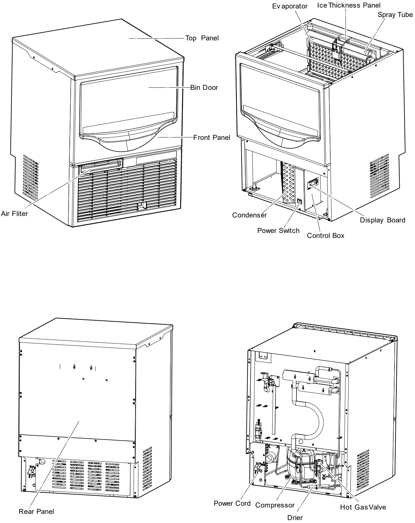
[d] SRM-125UB
