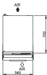
TOP SIDE
